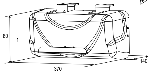
РАЗМЕРЫ(мм)
