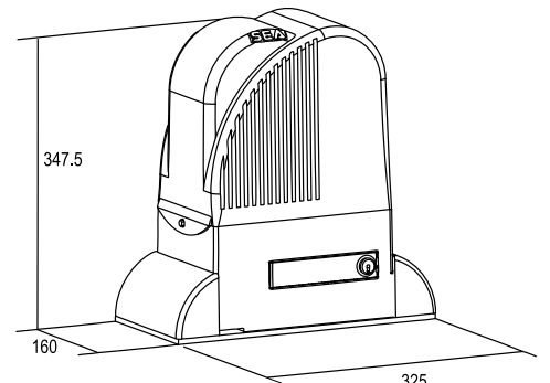
РАЗМЕРЫ (мм)
